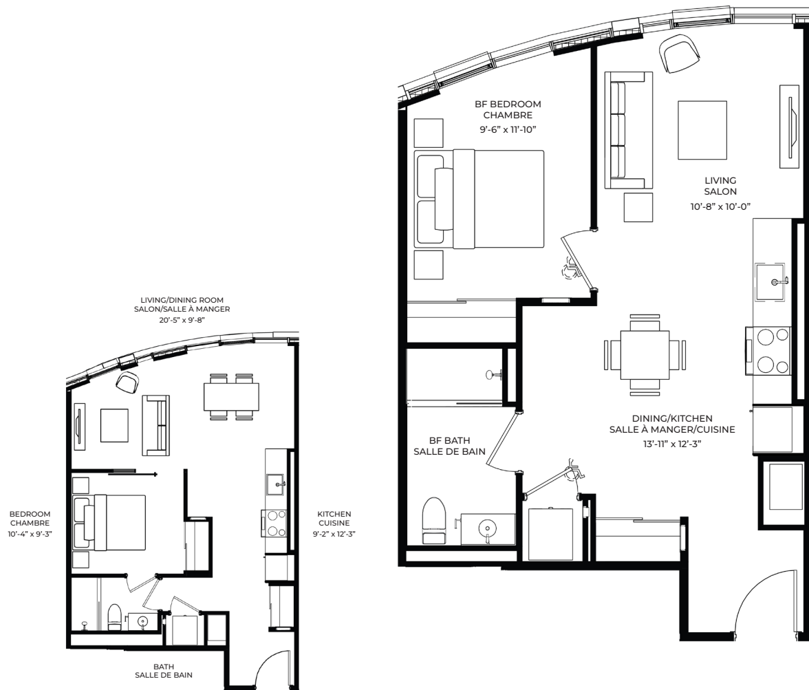
NON BF LAYOUT LEVEL 16-23
